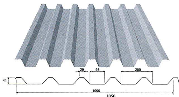
Till tak W-45/900
