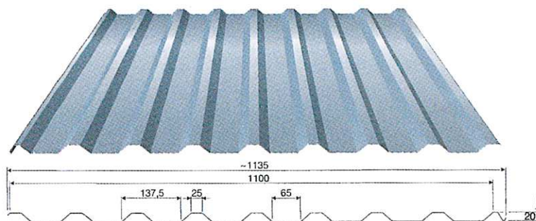
Till tak W-20/1100
